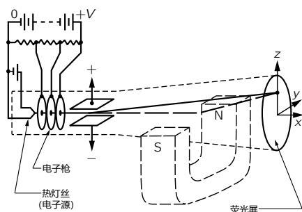
图 12.3: 电子束管
