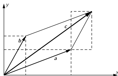
图 11.5: 矢量的加法
